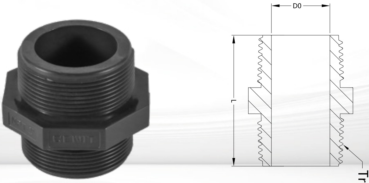
产品参数（美标 SCH80） SPECIFICATIONS(ASTM D2467 SCH80)
